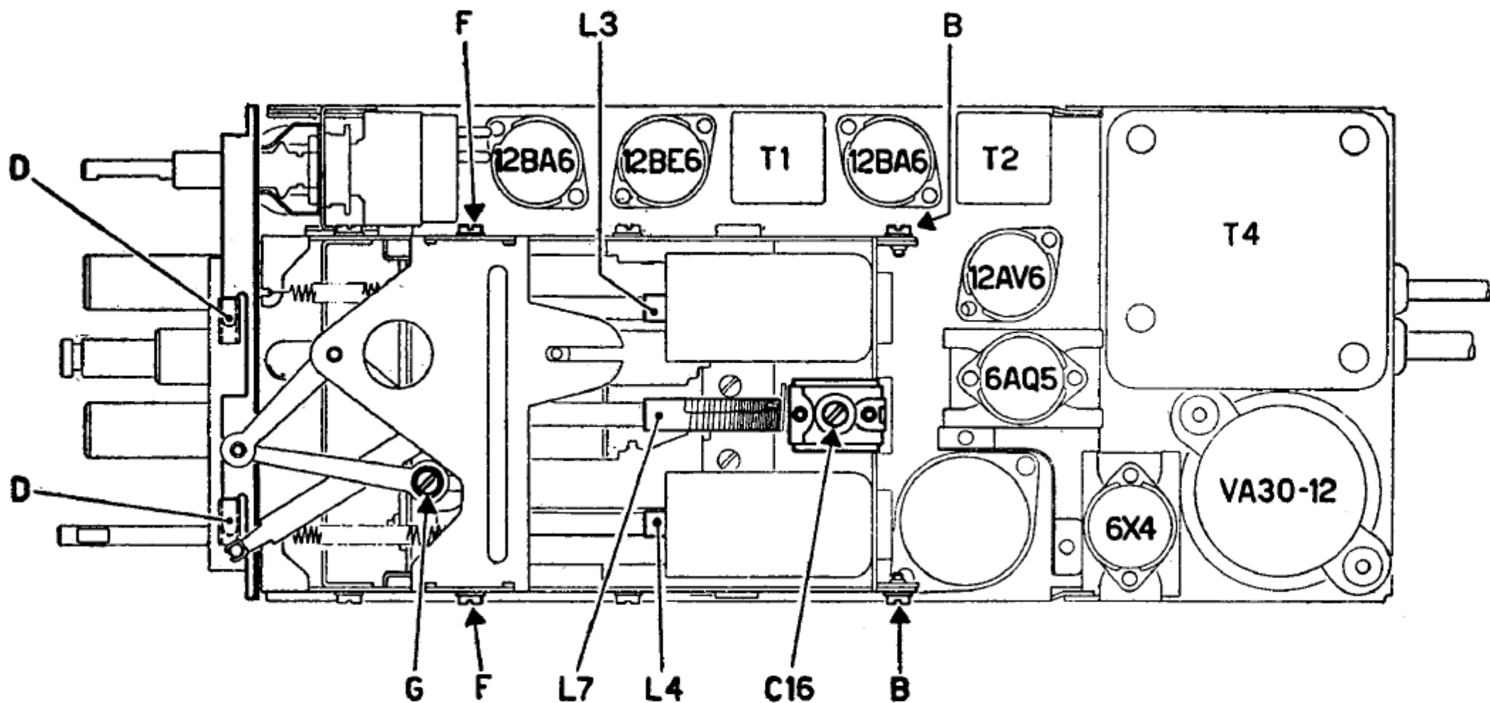
AUTOVOX RA 15 - Disposizione delle valvole e delle parti componenti.
